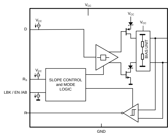
简化原理图
