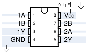
图 11-1. SN75451BD 布局
