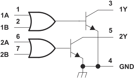
图 8-4. SNx5454B 逻辑图 ( 正逻辑 )
