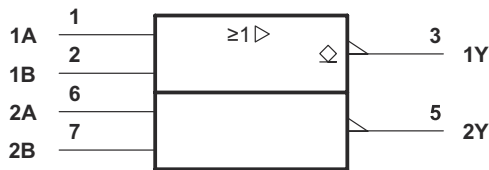
图 8-8. SNx5454B 逻辑符号
