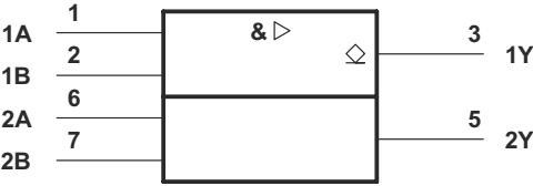
图 8-5. SNx5451B 逻辑符号
