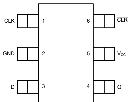
图 4-1. DBV 封装，6 引脚 SOT-23 (俯视图)
