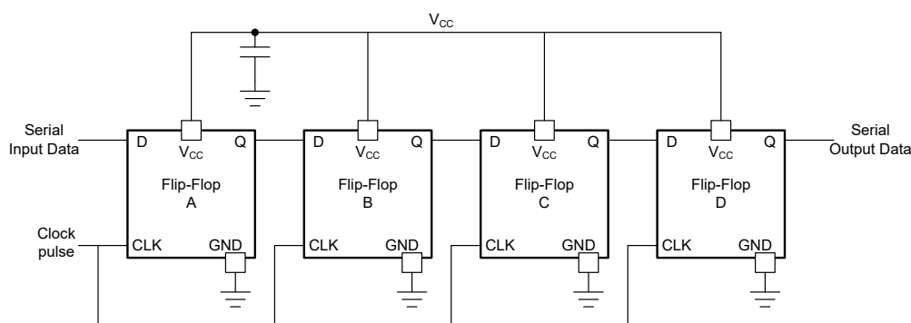
图 8-1. 4 位串行移位寄存器
