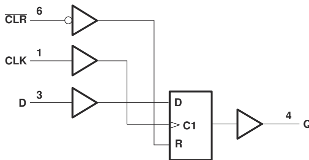
逻辑图
