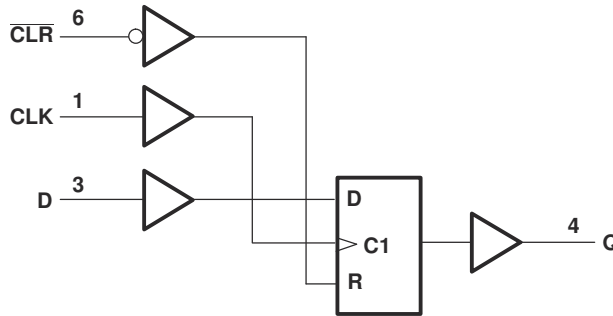
图 7-1. 逻辑图 (正逻辑)
