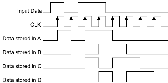
图 8-2. 应用时序图
