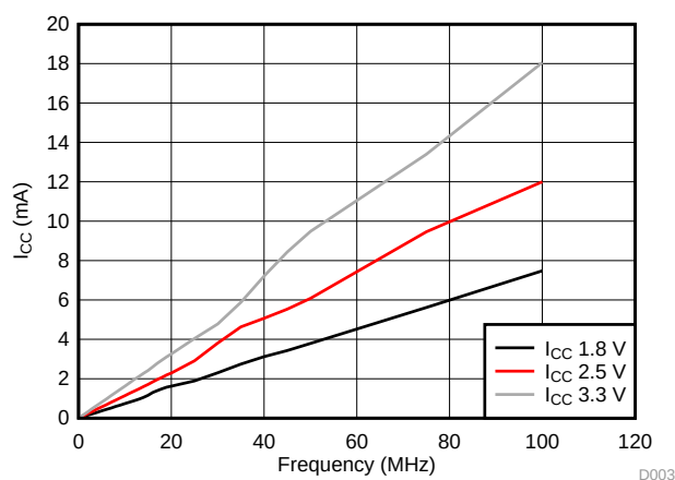
图 13. I_{CC} vs Frequency
