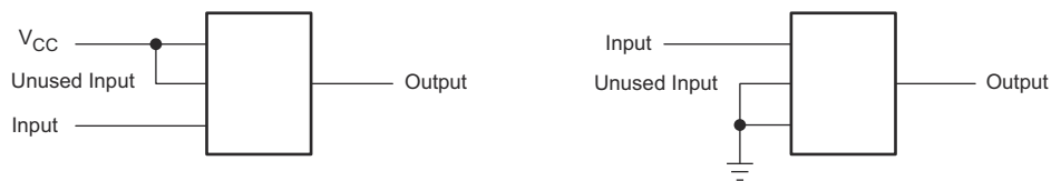
图 11-1. SNx4HC273 Layout
