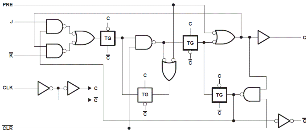
功能方框图
