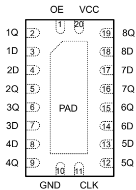
图 4-3. SN74AHCT374 RKS 封装 ( 顶视图 )
