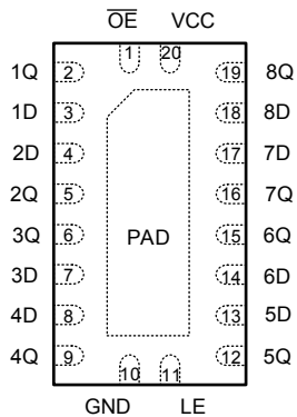
图 4-3. SN74AHCT373 RKS 封装 (顶视图)
