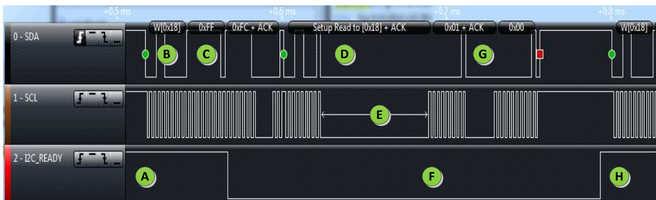
图 5-5. I 2 C 访问示例：读取状态寄存器地址 0xFFFC，响应为 0x00, 0x01 (Device_Ready = 1)
