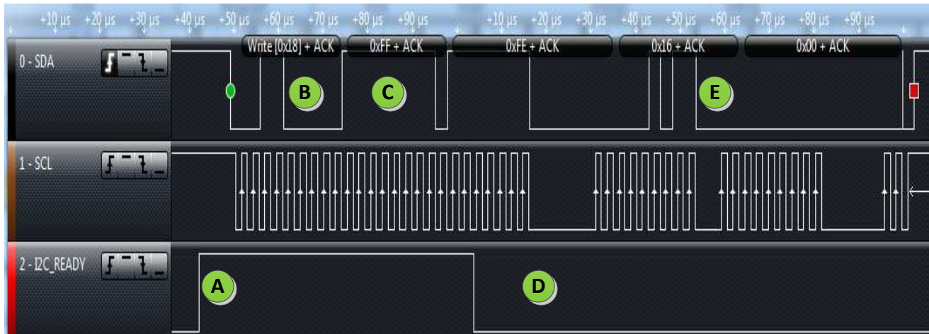
图 5-4. I 2 C 访问示例：写入控制寄存器地址 0xFFFE 使用 0x00, 0x16 (RF 启用 = 1)
