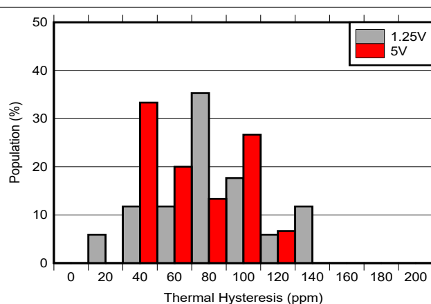
图 6-26. 热迟滞直方图 -40°C to 85°C 周期 1
