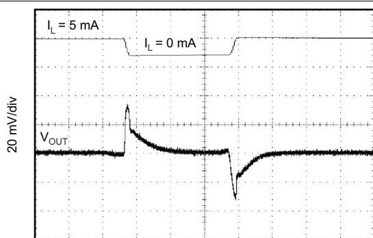
10 \mu\text{s}/\text{div} C_L = 0 图 6-46. 0mA 至 5mA 负载瞬态
