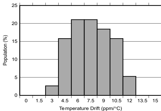
图 6-2. 温漂直方图 ( -40°C 至 +85°C )
