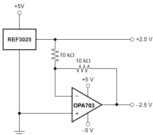
图 7-3. REF3025 与 OPA703 结合使用可产生正和负基准电压。
