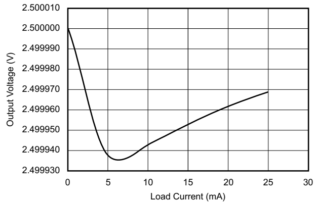
图 6-41. 输出电压与负载电流间的关系
