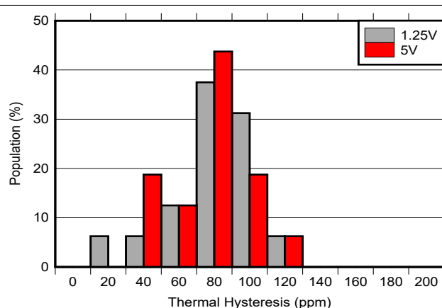
图 6-28. 热迟滞直方图 0°C to 70°C 周期 1
