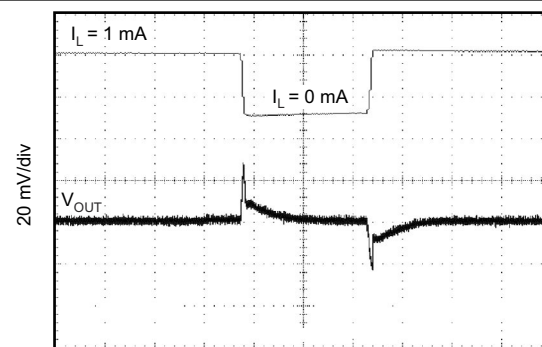
10 \mu\text{s}/\text{div} C_L = 0 图 6-45. 0mA 至 1mA 负载瞬态
