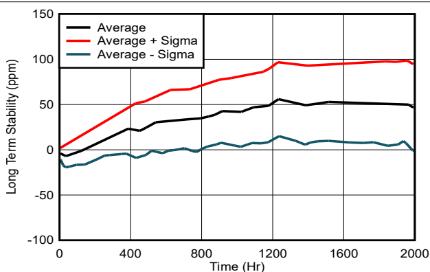
图 6-23. 长期稳定性: 0 到 2000 小时
