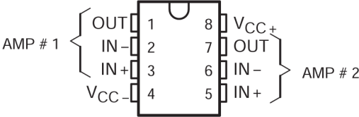
D 或 P 封装，8 引脚 SOIC 或 PDIP ( 顶视图 )
