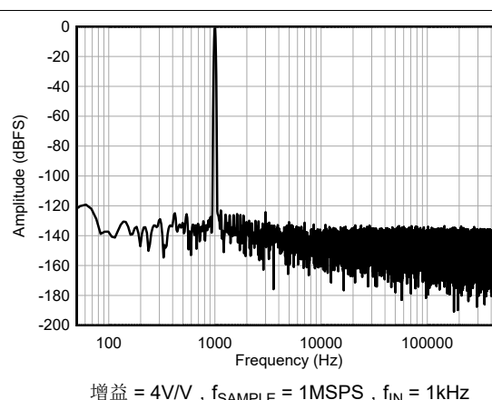
图 9-11. 使用 ADS8900B 的性能 FFT 图
