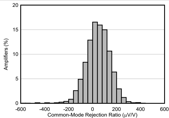
图 7-21. CMRR 分布
