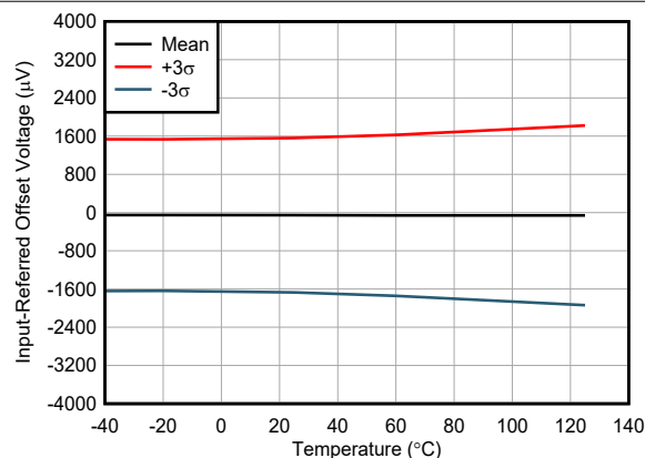
图 7-17. 失调电压 (RTI) 与温度间的关系
