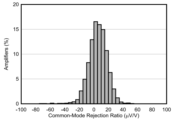
图 7-22. CMRR 分布
