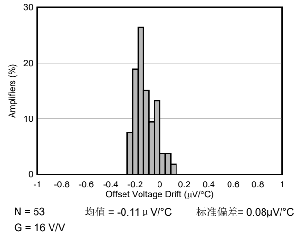
图 7-2. 失调电压漂移 (RTI) 的分布
