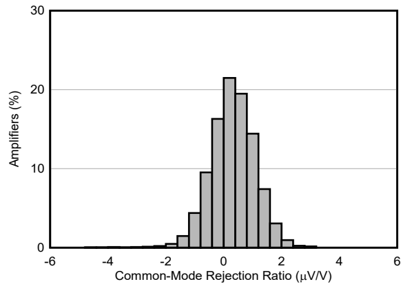
图 7-21. CMRR 分布
