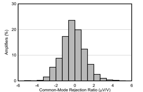
图 6-16. CMRR 分布
