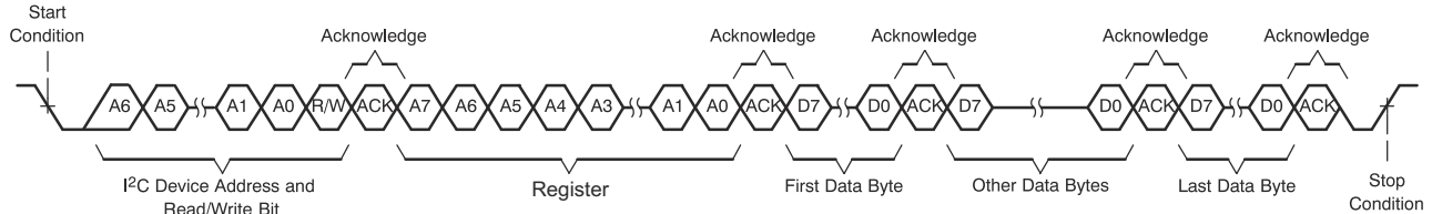
图 7-65. I 2 C Multiple-Byte Write Transfer
