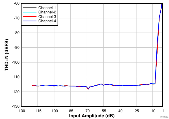
图 8-3. THD+N vs Input Amplitude
