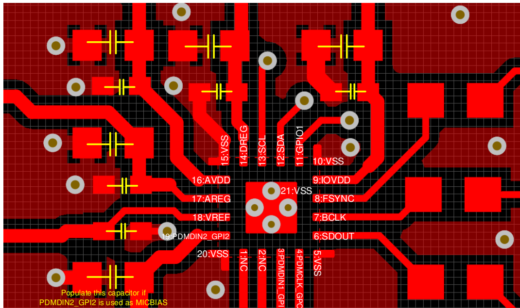
图 10-1. Layout Example
