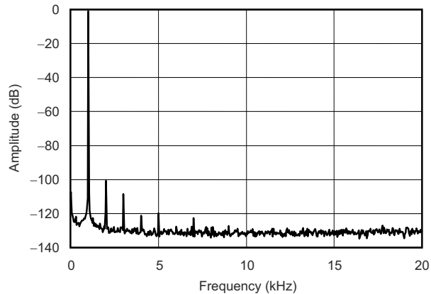
图 8-4. Output Spectrum
