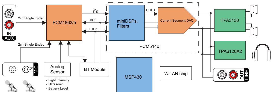
简化系统图
