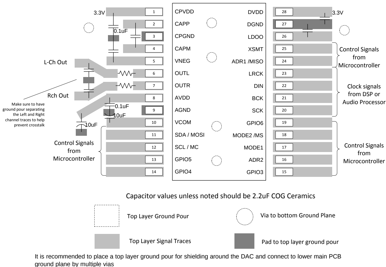
图 87. PCM514x Layout Example
