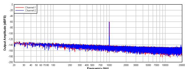
图 9-6. PCM1821-Q1: FFT With a - 60-dBr Input
