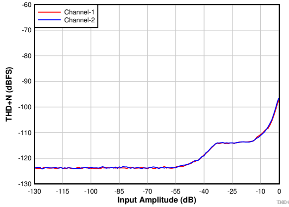
图 7-1. PCM1820-Q1: THD+N vs Input Amplitude With DRE Enabled
