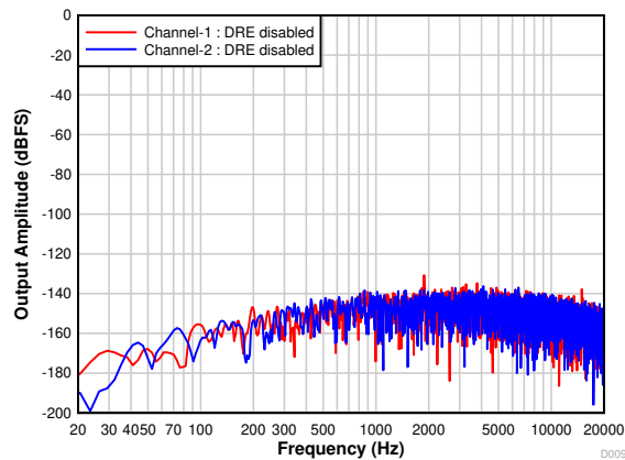
图 7-9. PCM1820-Q1: FFT With Idle Input and DRE Disabled
