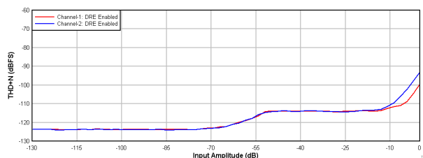
图 9-3. PCM1820-Q1: THD+N vs Input Amplitude With DRE Enabled
