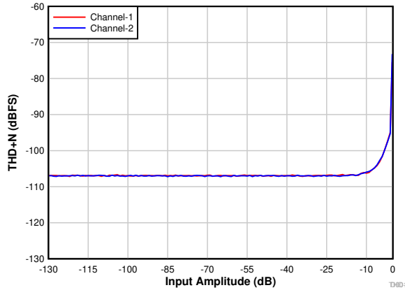
图 7-13. PCM1821-Q1: THD+N vs Input Amplitude
