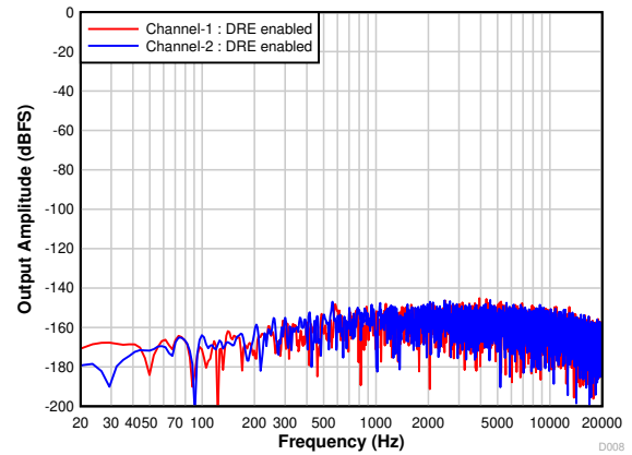
图 7-8. PCM1820-Q1: FFT With Idle Input and DRE Enabled
