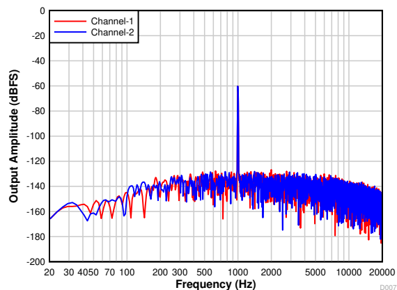
图 7-19. PCM1821-Q1: FFT With a -60-dBr Input and DRE Enabled
