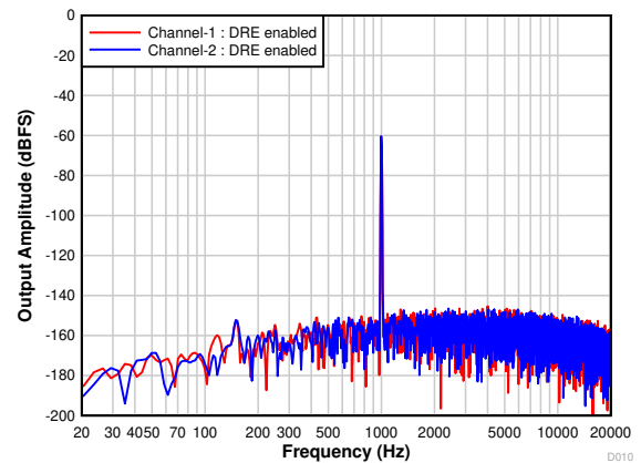
图 7-10. PCM1820-Q1: FFT With a -60-dBr Input and DRE Enabled
