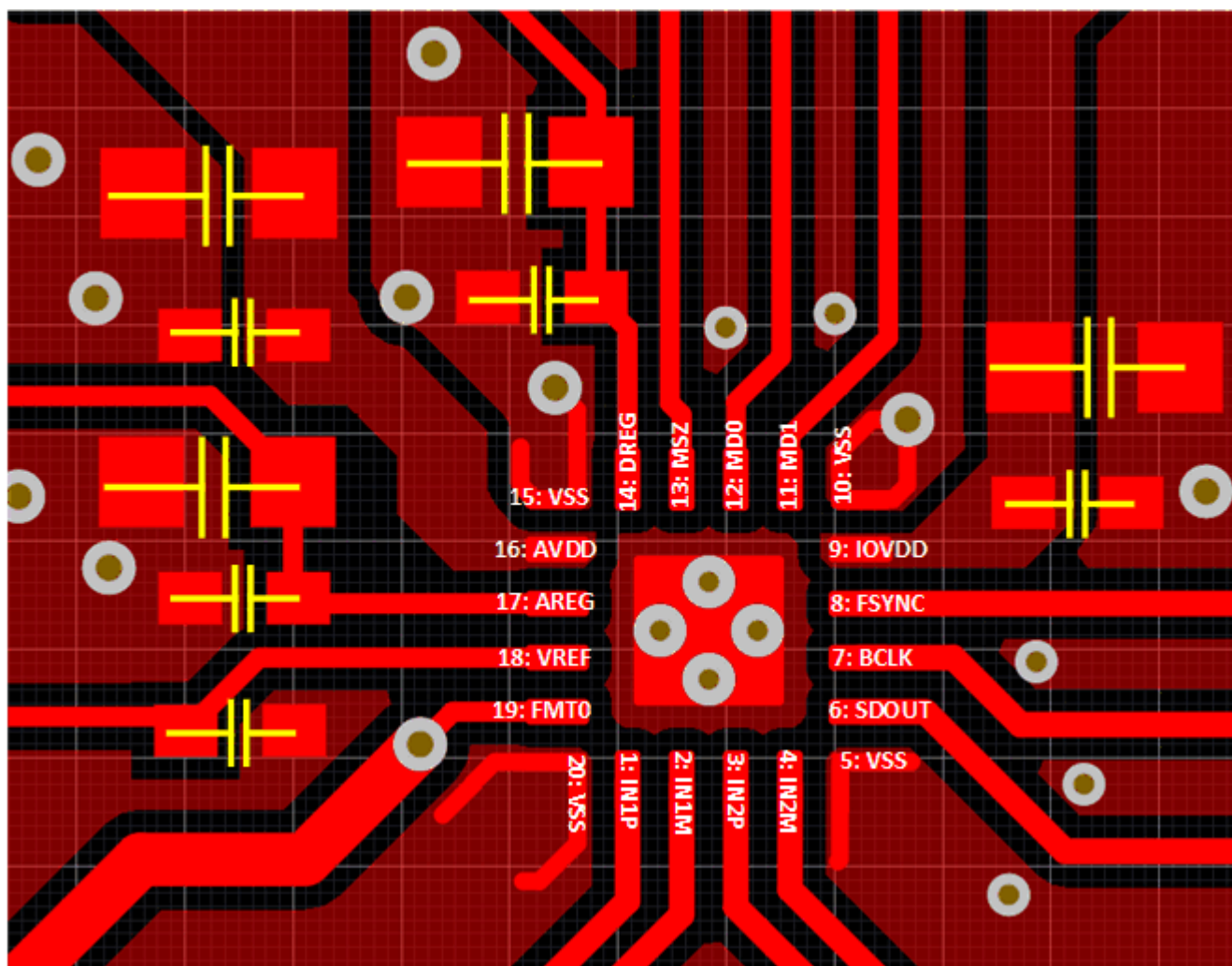
图 11-1. Example Layout
