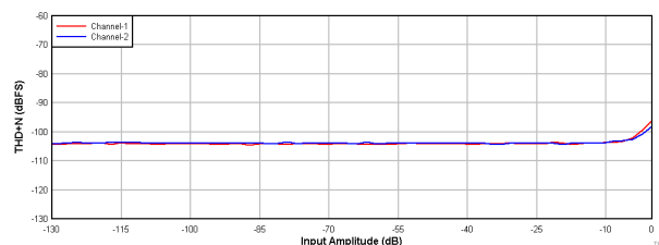
图 9-7. PCM1821-Q1: THD+N vs Input Amplitude
