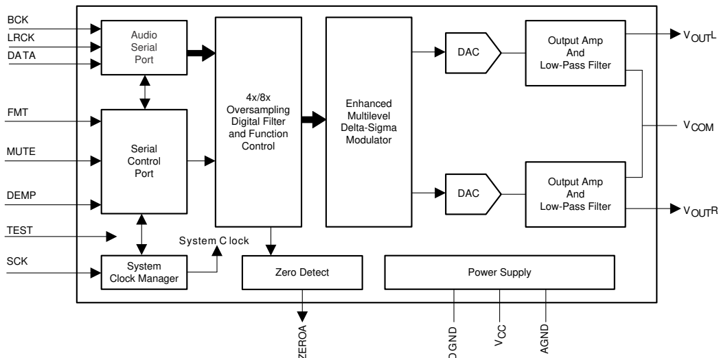
功能方框图
