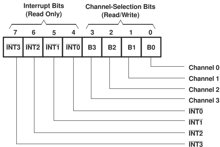
图 8-8. Control Register
