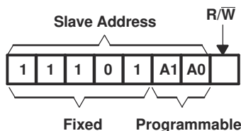
图 8-6. Pca9539 Address
