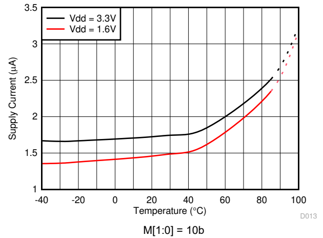
图 5-19. 电源电流与温度间的关系 (3 级)
