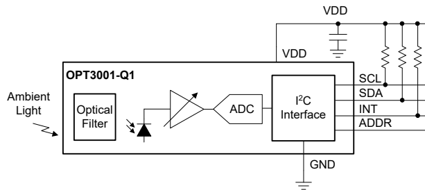
方框图
