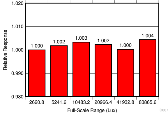
图 5-8. 满标量程匹配 (最高的 6 个量程)
