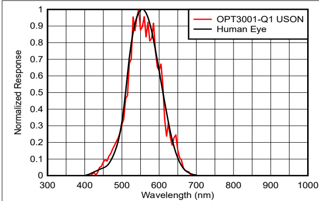
图 5-2. 光谱响应与波长间的关系
