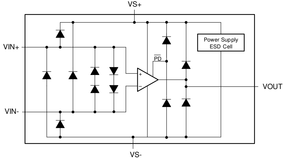
图 7-1. 内部 ESD 保护
