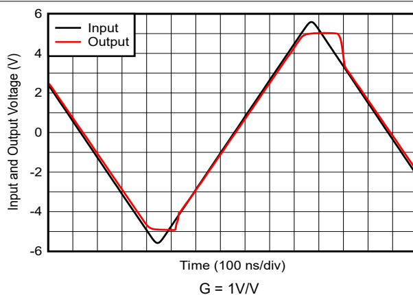
图 6-10. 输入过驱恢复
