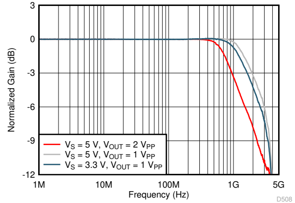
图 6-8. 大信号频率响应与电压电源间的关系
