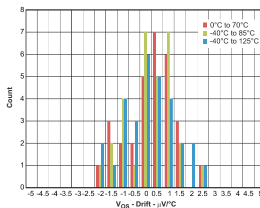
图 7-22. Input Offset Voltage Drift
