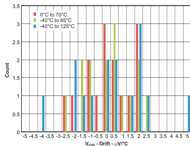
图 7-23. Input Offset Voltage Drift
