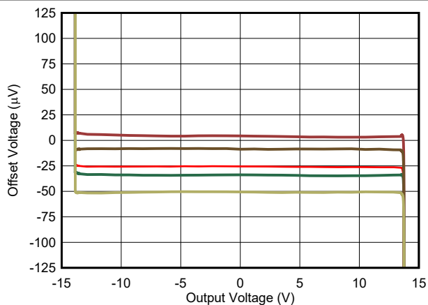
图 6-12. 失调电压与输出电压间的关系
