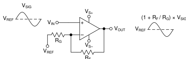
图 7-1. Noninverting Amplifier
