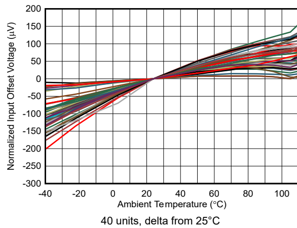
图 6-25. Input Offset Voltage vs Temperature
