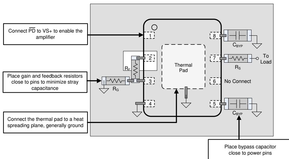
图 8-6. Layout Recommendation
