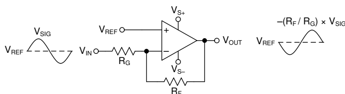
图 7-2. Inverting Amplifier
