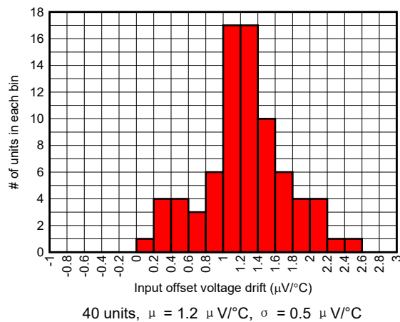
图 6-27. Input Offset Voltage Drift Histogram
