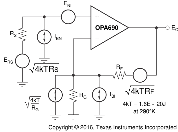
图 8-4. Op Amp Noise Analysis Model
