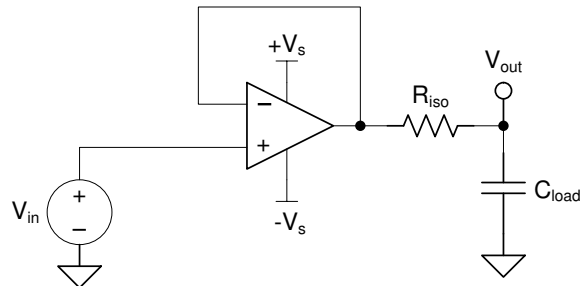
图 6-7. 使用 OPA992 扩展容性负载驱动
