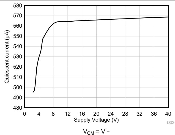
图 6-23. 静态电流与电源电压间的关系
