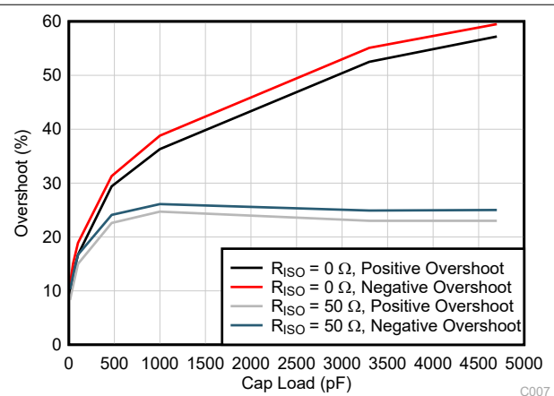
图 7-6. 小信号过冲与容性负载之间的关系 (10mV 输出阶跃, G = -1 )
