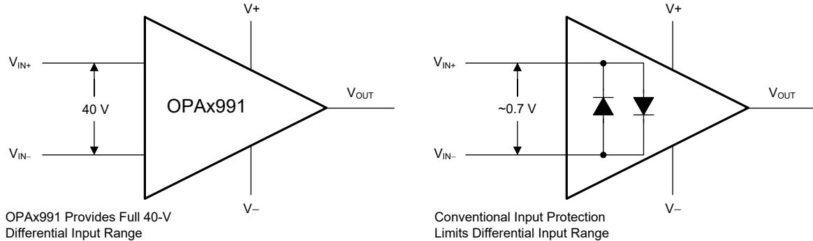
图 7-1. OPA x 991 输入保护不限制差分输入能力
