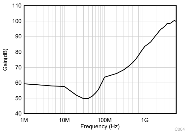
图 7-3. EMIRR 测试
