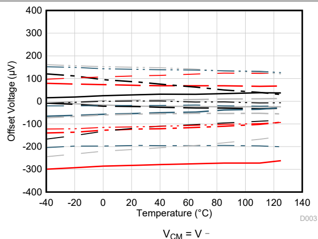
图 6-4. 失调电压与温度间的关系
