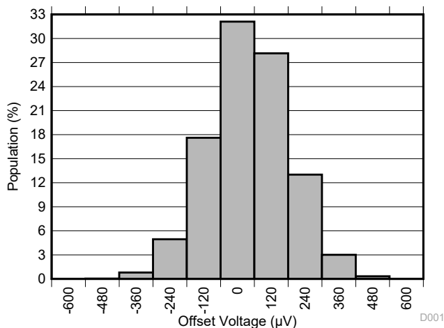
图 6-1. 失调电压生产分配
