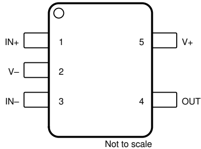
图 5-2. OPA991 DCK 封装 5 引脚 SC70 (顶视图)
