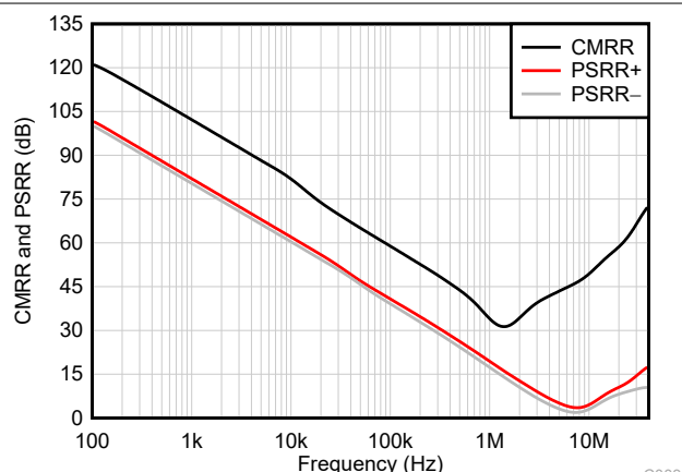
图 6-16. CMRR 和 PSRR 与频率间的关系
