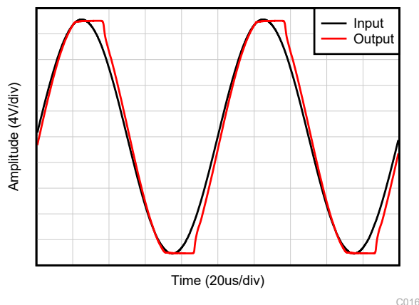
图 7-9. 无相位反转
