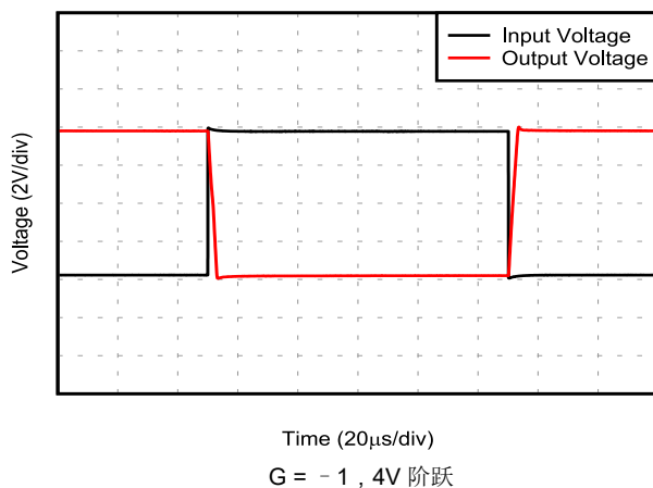
图 5-38. 大信号阶跃响应
