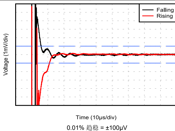
图 5-39. 趋稳时间
