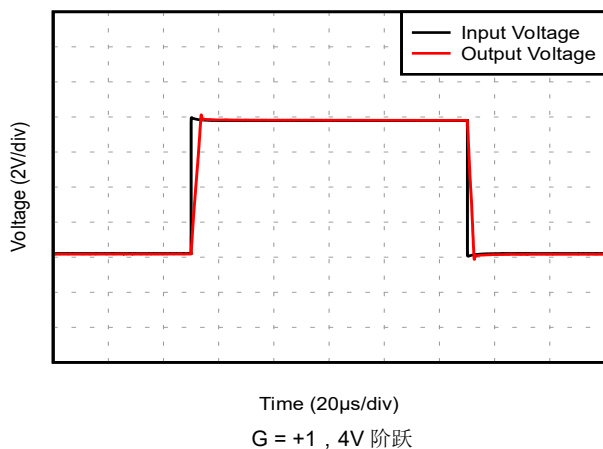
图 5-37. 大信号阶跃响应
