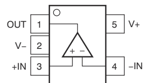
图 4-2. OPA171 DBV 封装：5 引脚 SOT-23（顶视图）
