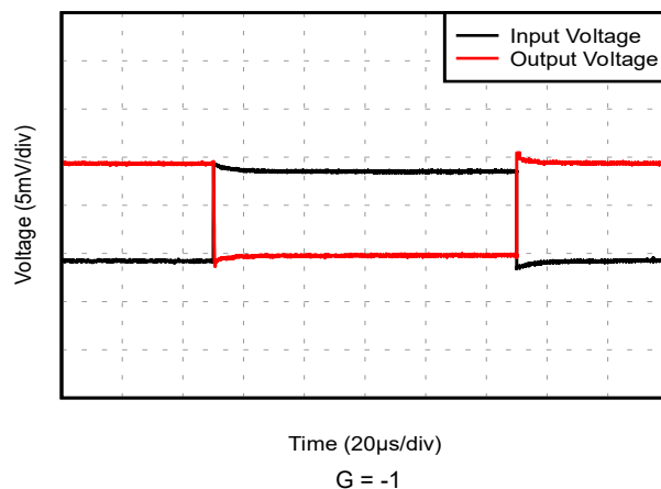
图 5-36. 小信号阶跃响应
