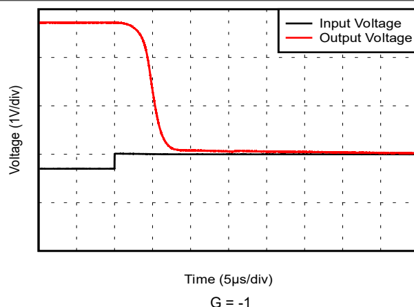
图 5-34. 过载恢复
