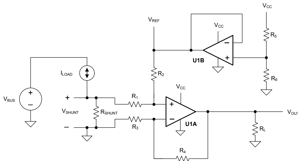
图 7-1. 双向电流感应原理图
