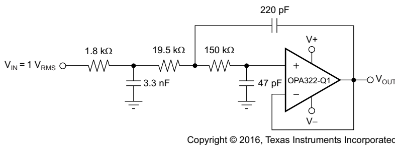
图 34. OPAx322-Q1 配置为三极 20kHz Sallen-Key 滤波器
