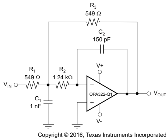
图 33. 二阶巴特沃斯 500kHz 低通滤波器
