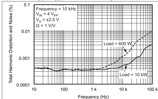
图 19. THD+N 与频率间的关系
