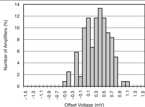
图 7. 失调电压产生直方图
