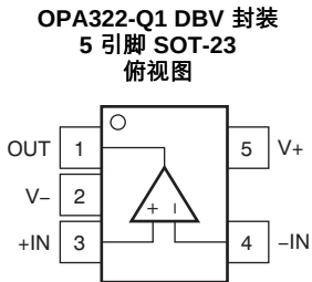
引脚功能：OPA322-Q1
