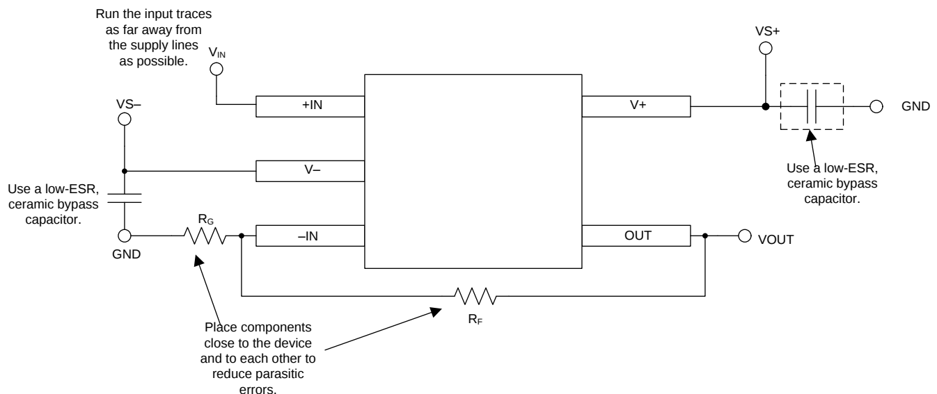
图 45. 同相配置的运算放大器电路板布局
