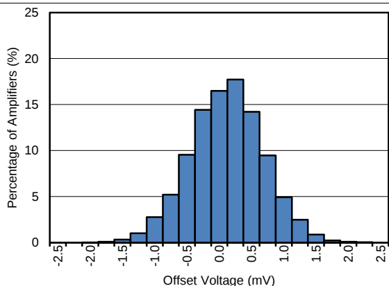
根据 12551 个放大器得出的分布图
