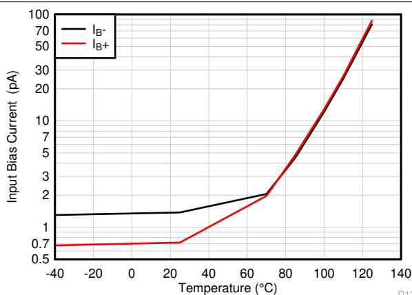
图 6-13. I_B 与温度间的关系
