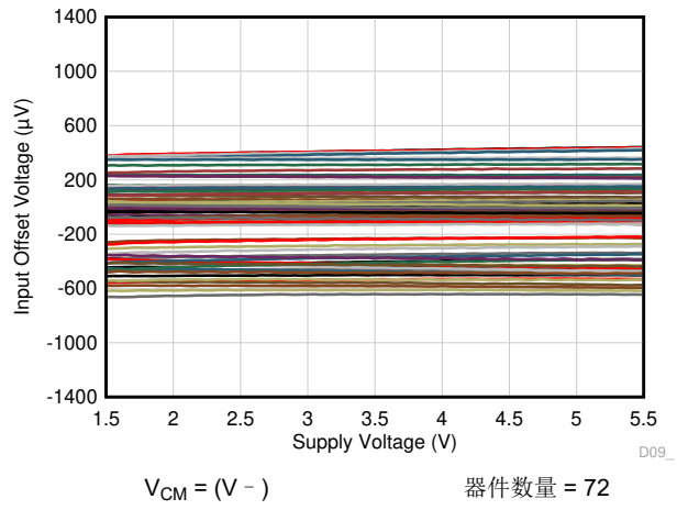
图 6-12. 失调电压与电源电压间的关系
