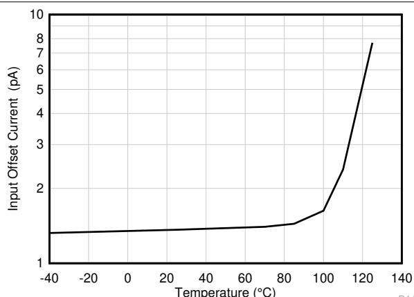
图 6-14. I_{OS} 与温度间的关系
