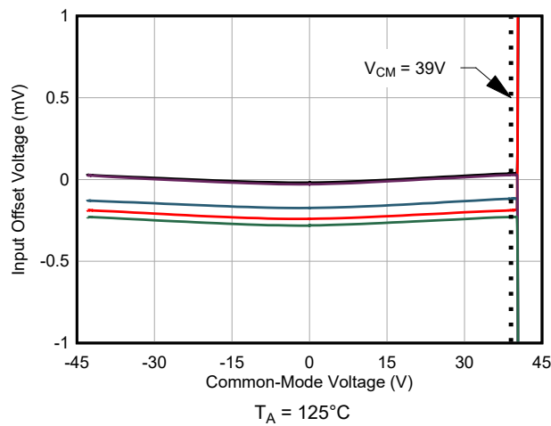
图 5-5. 输入失调电压与共模电压间的关系
