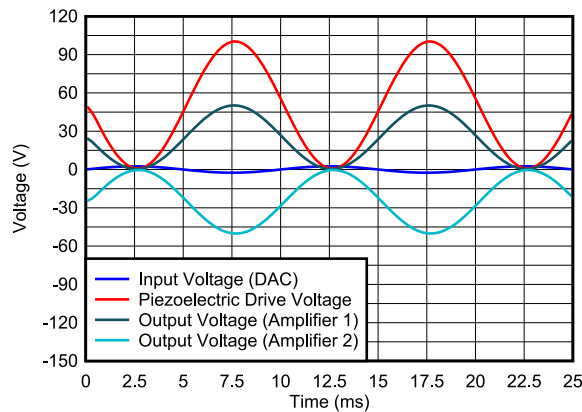
图 7-2. 压电式驱动器输出电压
