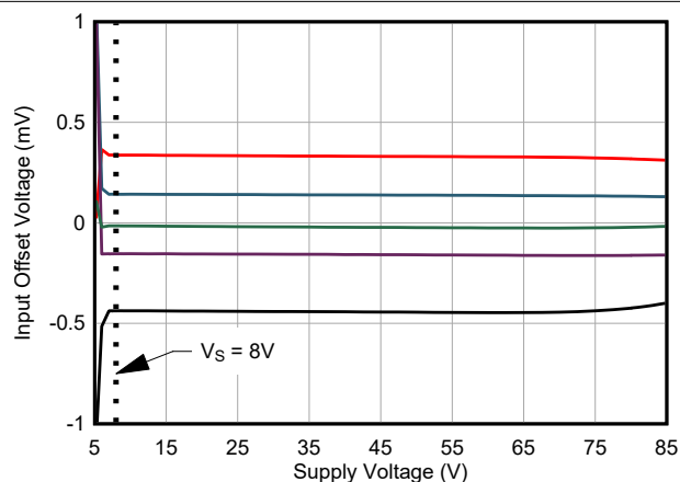
图 5-9. 失调电压与电源电压间的关系
