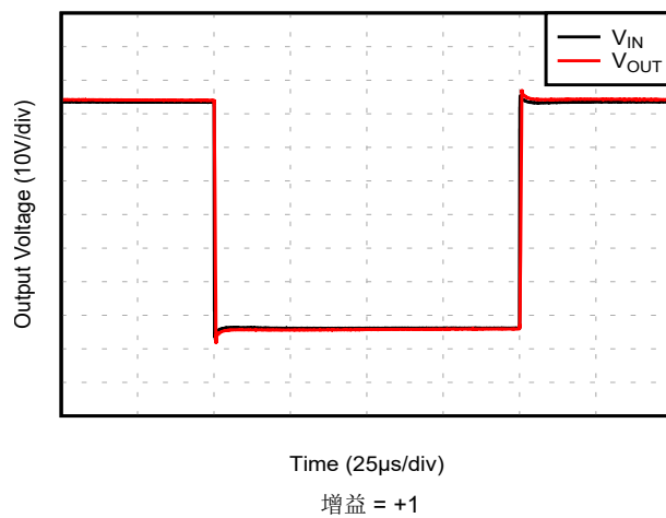
图 5-34. 大信号阶跃响应
