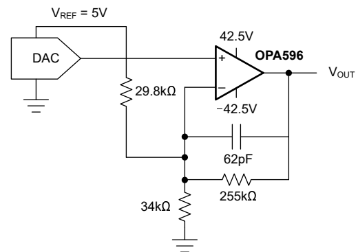
具有增益的 DAC 输出缓冲器
