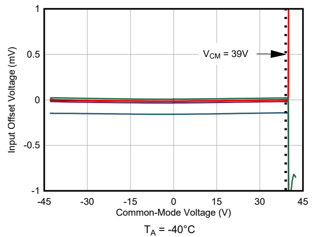
图 5-6. 输入失调电压与共模电压间的关系
