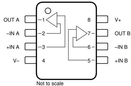
图 4-2. OPA2596 D 封装，8 引脚 SOIC 和 DGK 封装，8 引脚 VSSOP (顶视图)
