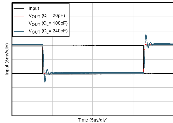
图 5-32. 负过载恢复
