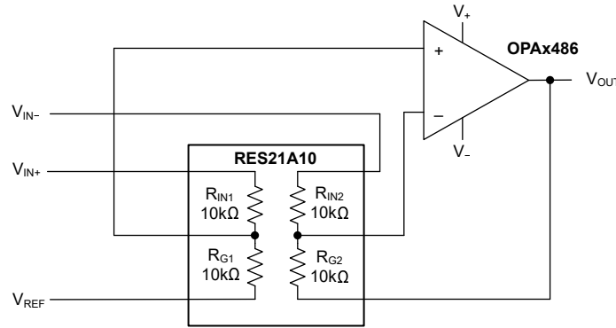
图 7-7. 差分放大器
