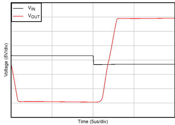
图 5-32. 负过载恢复
