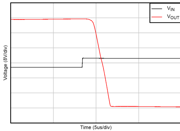
图 5-31. 正过载恢复
