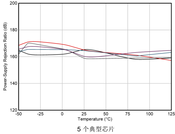
图 5-19. PSRR 与温度间的关系
