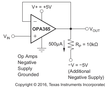
图 8-4. 摆动到接地
