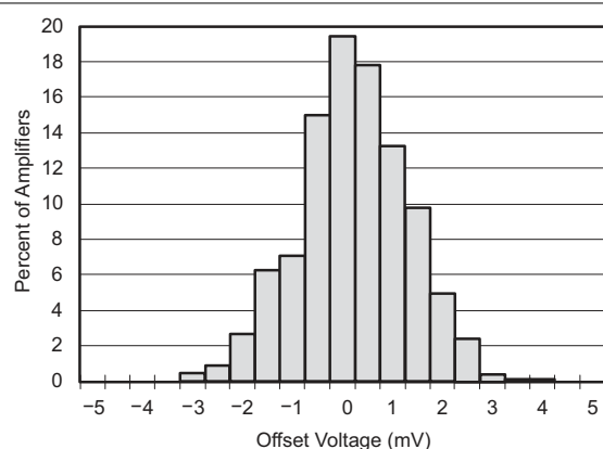
图 5-30. 失调电压产生分布
