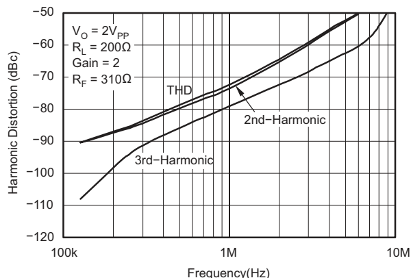
图 5-11. 谐波失真与频率间的关系
