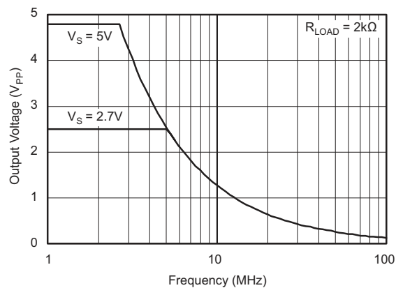
图 5-24. 最大输出电压与频率间的关系
