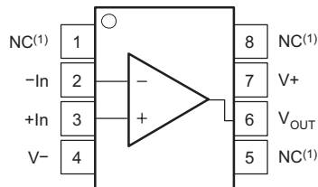
图 4-4. OPA301 , SO-8 封装 , 8 引脚 ( 顶视图 )
