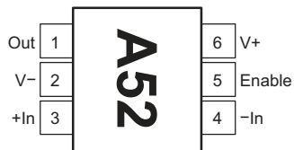
图 4-1. OPA300 , SOT 23 封装 6 引脚 ( 顶视图 )
