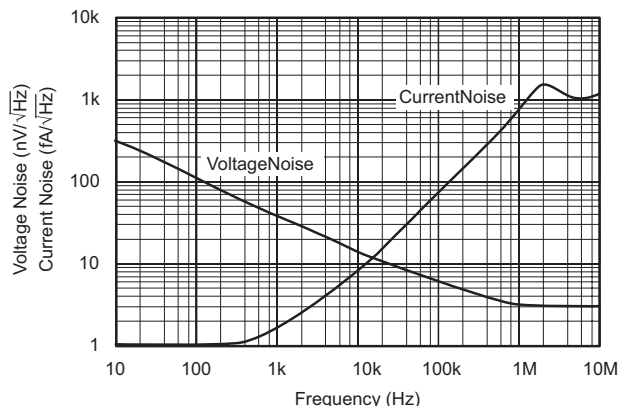
图 5-12. 输入电压和电流噪声频谱密度与频率间的关系
