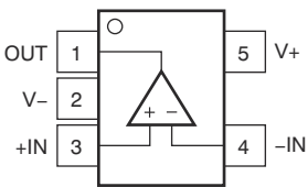
图 6-2. OPA182 DBV ( 5 引脚 SOT-23 ) 封装，顶视图
