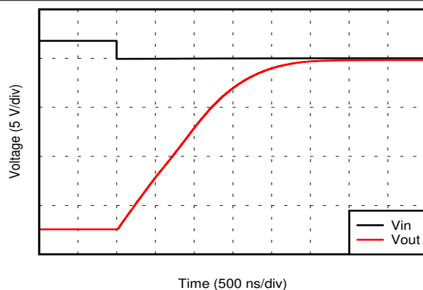
图 7-27. 无相位反转
