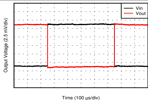
反相配置
