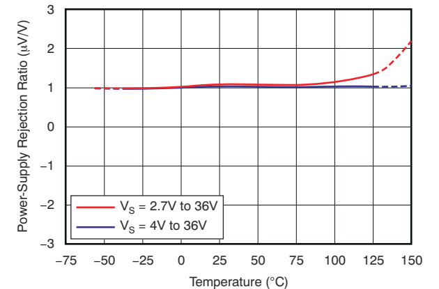
图 5-12. PSRR 与温度间的关系
