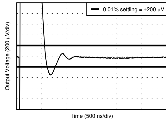
图 6-38. 大信号阶跃响应
