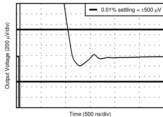
图 6-40. 0.01% 稳定时间
