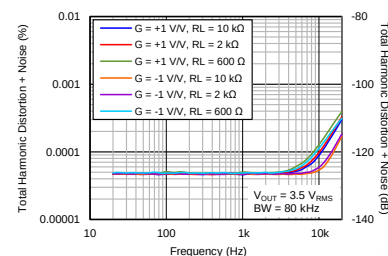
出色的总谐波失真 (THD) 性能
