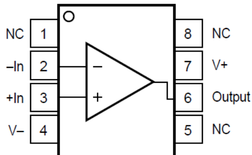
图 4-2. OPA137、SO-8
