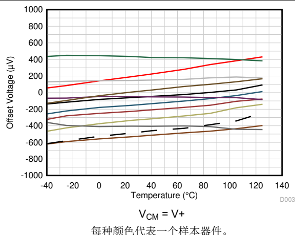
图 5-21. 偏移电压与温度间的关系 (新裸片)
