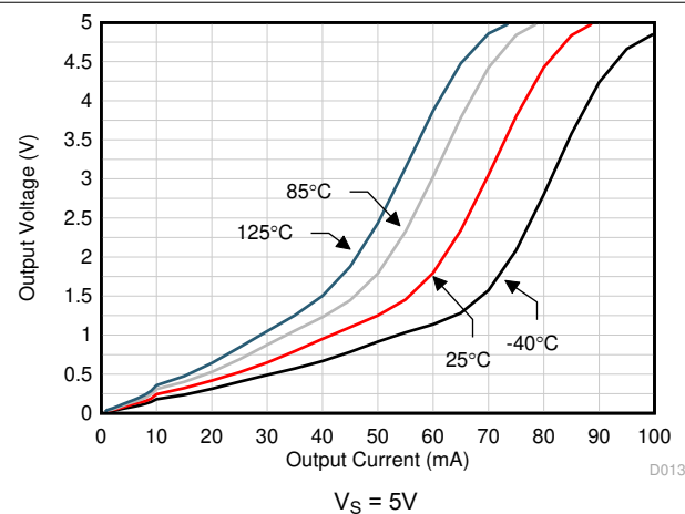
图 5-35. 输出电压摆幅与输出电流 (灌电流) 间的关系 (新裸片)
