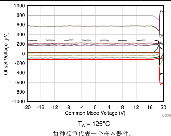
图 5-25. 偏移电压与共模电压间的关系 (新裸片)
