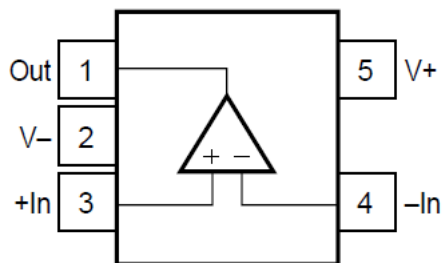
图 4-1. OPA137 SOT-23-5
