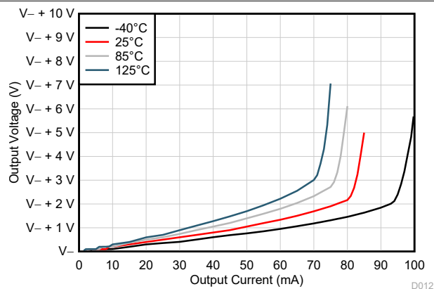
图 5-33. 输出电压摆幅与输出电流 (灌电流) 间的关系 (新裸片)
