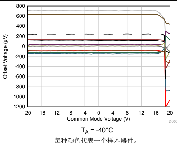
图 5-26. 偏移电压与共模电压间的关系 (新裸片)
