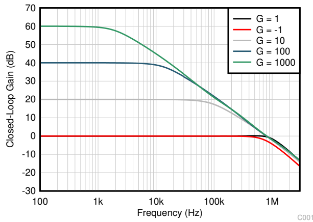
图 5-29. 闭环增益与频率间的关系 (新裸片)
