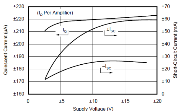
图 5-10. 静态电流和短路电流与电源电压间的关系 (旧裸片)
