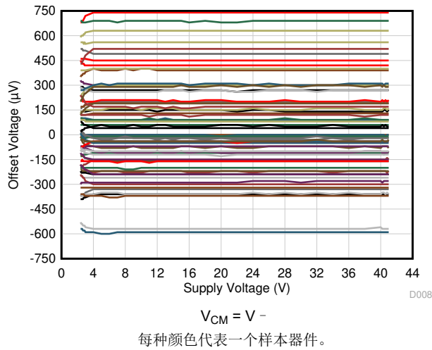
图 5-27. 偏移电压与电源电压间的关系 (新裸片)
