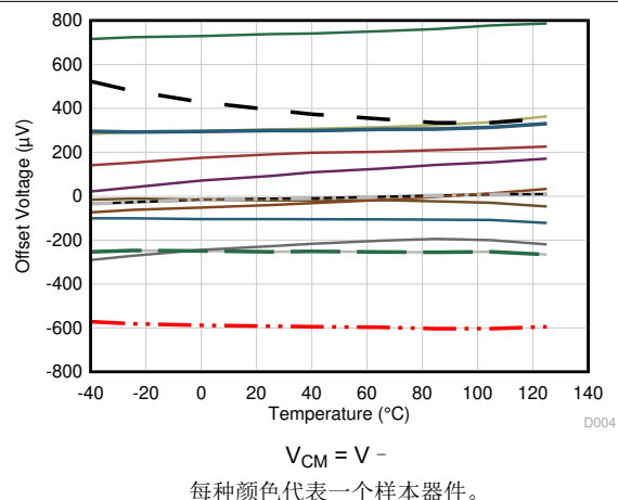
图 5-22. 偏移电压与温度间的关系 (新裸片)
