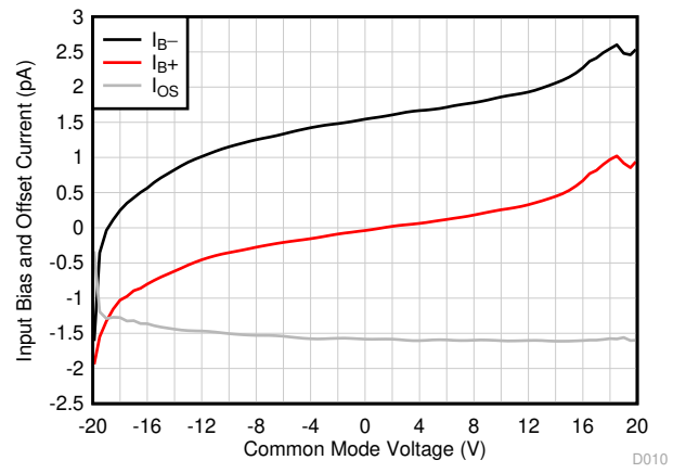
图 5-30. 输入偏置电流与共模电压间的关系 (新裸片)
