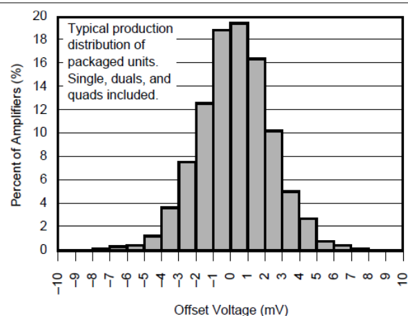
图 5-13. 偏移电压产生分布图 (旧裸片)
