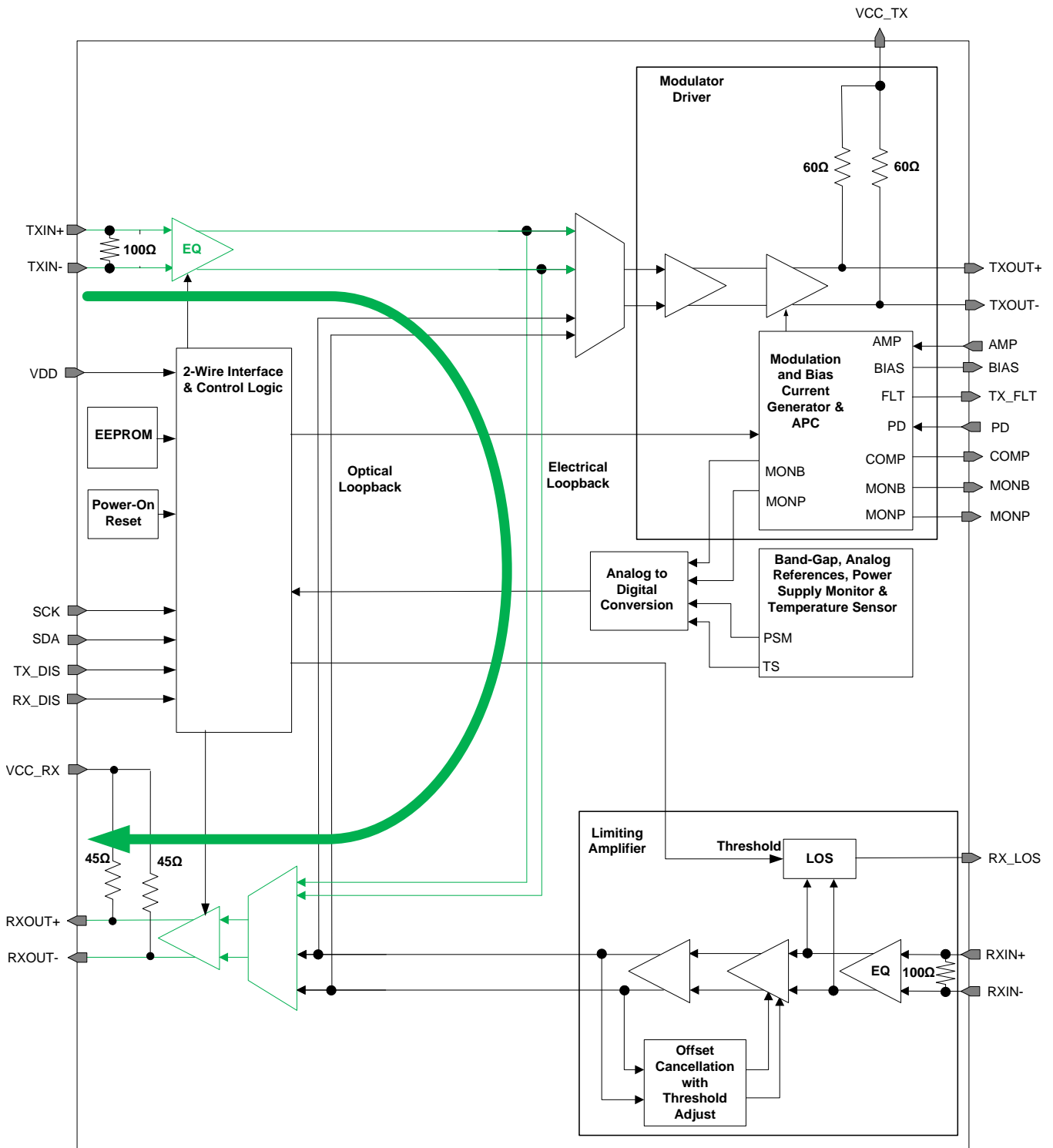
图 35. Electrical Loopback
