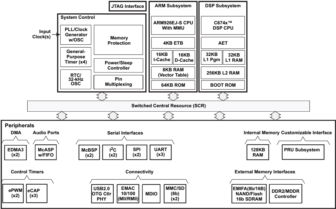
图 1-1. 功能框图
