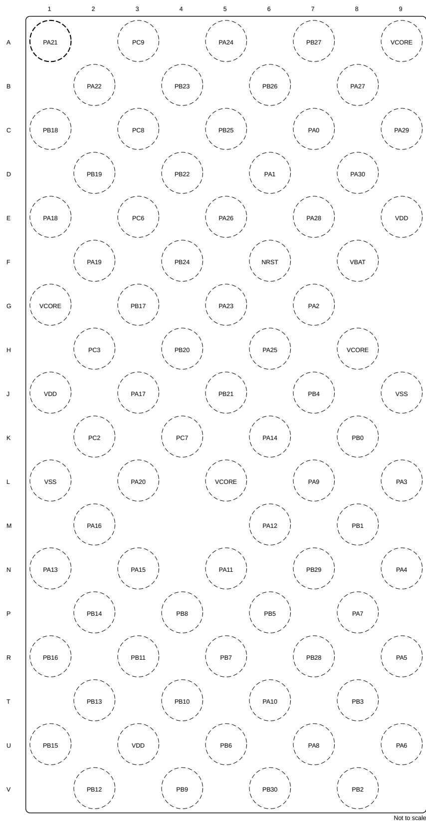
图 6-6. 79 引脚 YSG (3.6mm x 3.24mm) ( 0.35mm 间距 ) (WCSP) 封装图 ( 顶视图 )
