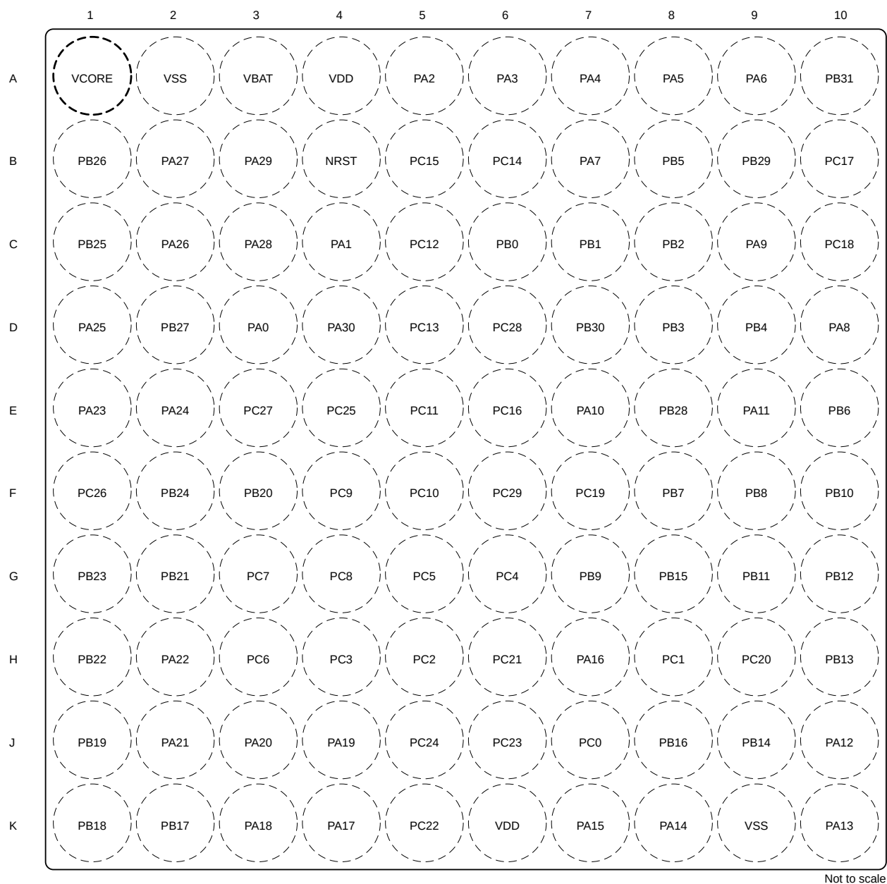
图 6-1. 100 引脚 ZAW (9mm x 9mm) ( 0.8mm 间距 ) (NFBGA) 封装图 ( 顶视图 )
