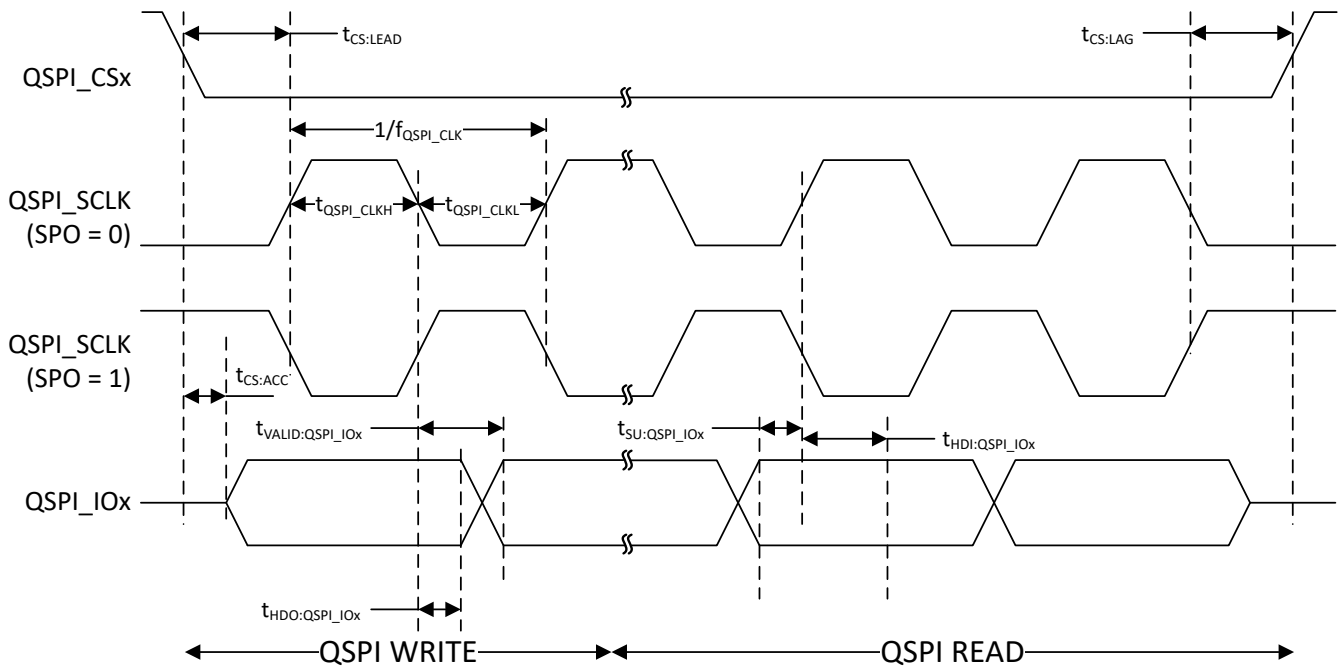
图 7-6. QSPI 时序图 - 控制器模式
