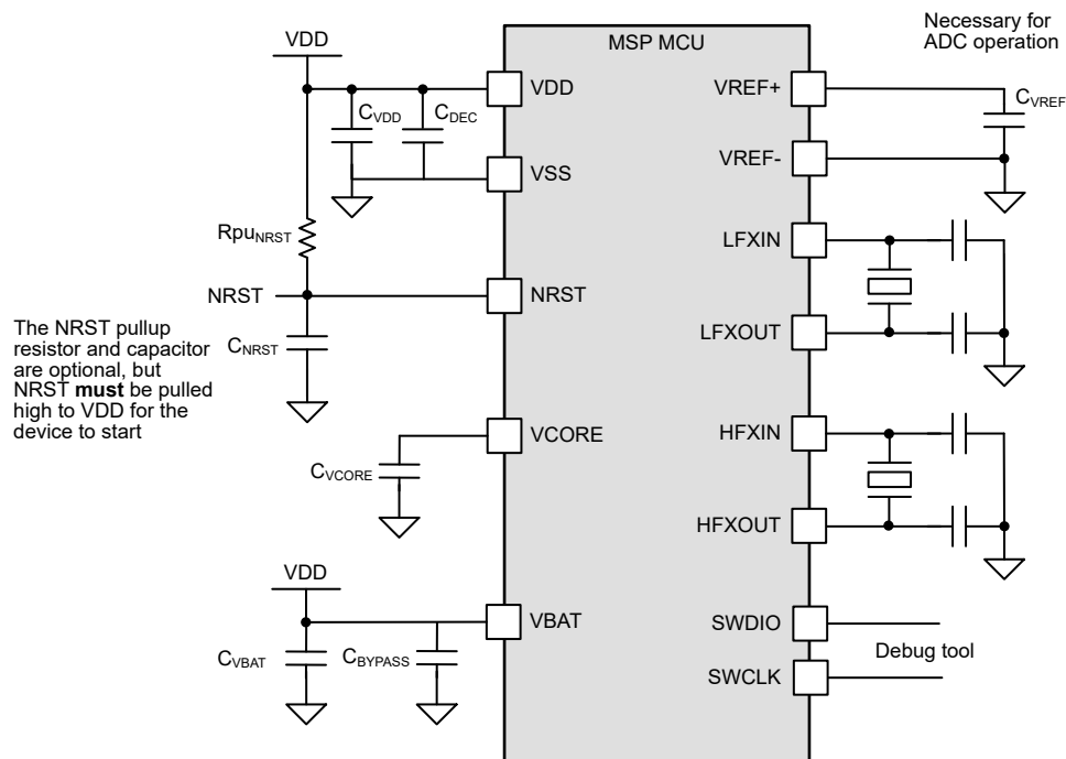
图 9-1. 基本应用原理图
