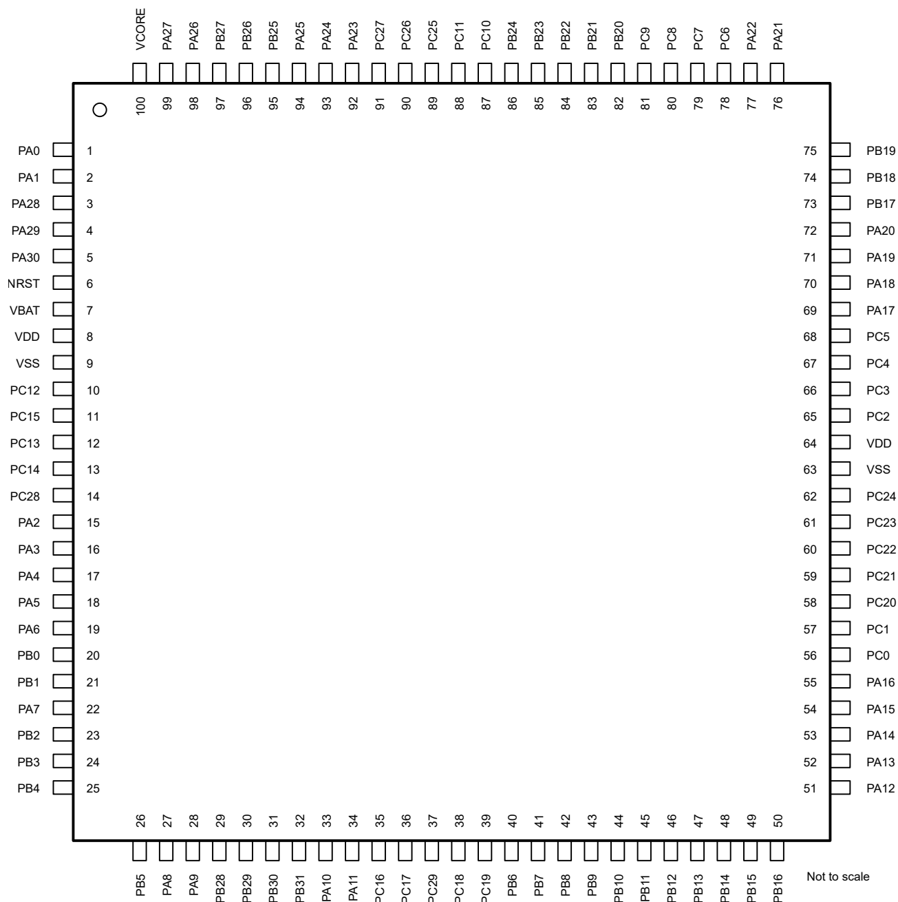
图 6-2. 100 引脚 PFA (14mm x 14mm) ( 0.4mm 间距 ) 和 PZ (16mm x 16mm) ( 0.5mm 间距 ) (LQFP) 封装图 ( 顶视图 )
