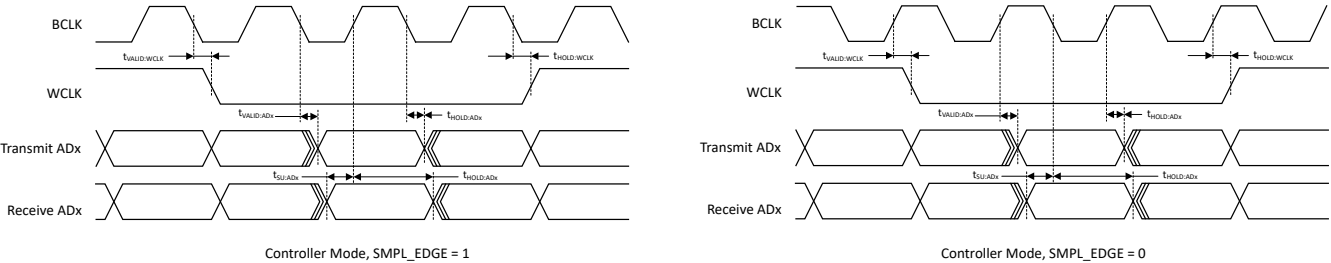
图 7-7. I2S/TDM 时序图 - 控制器模式
