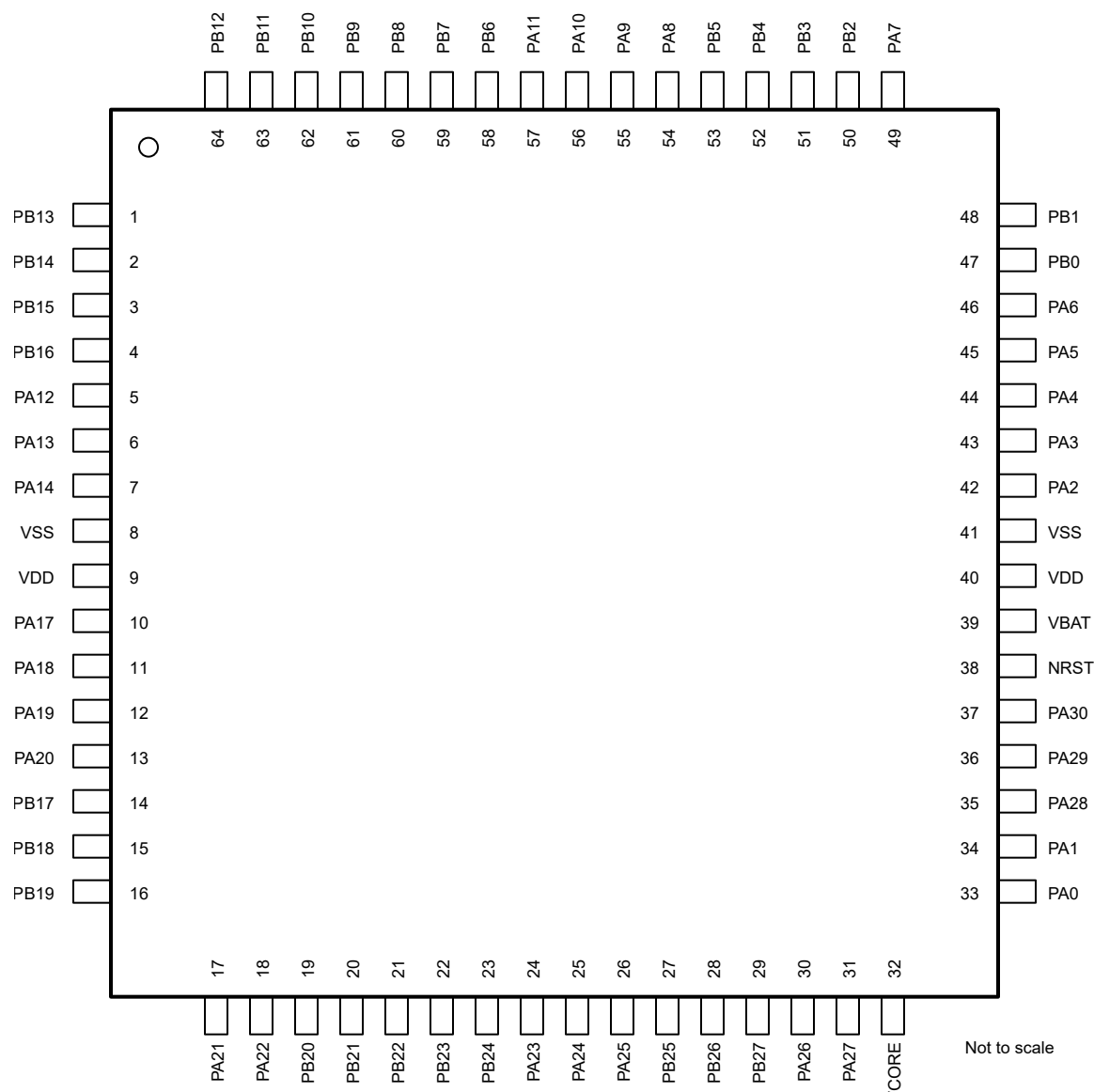
图 6-4. 64 引脚 PM (12mm x 12mm) ( 0.5mm 间距 ) (LQFP) 封装图 ( 顶视图 )
