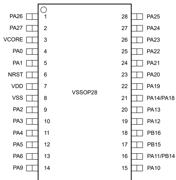
图 6-6. 28 引脚 DGS28 (VSSOP) 封装
