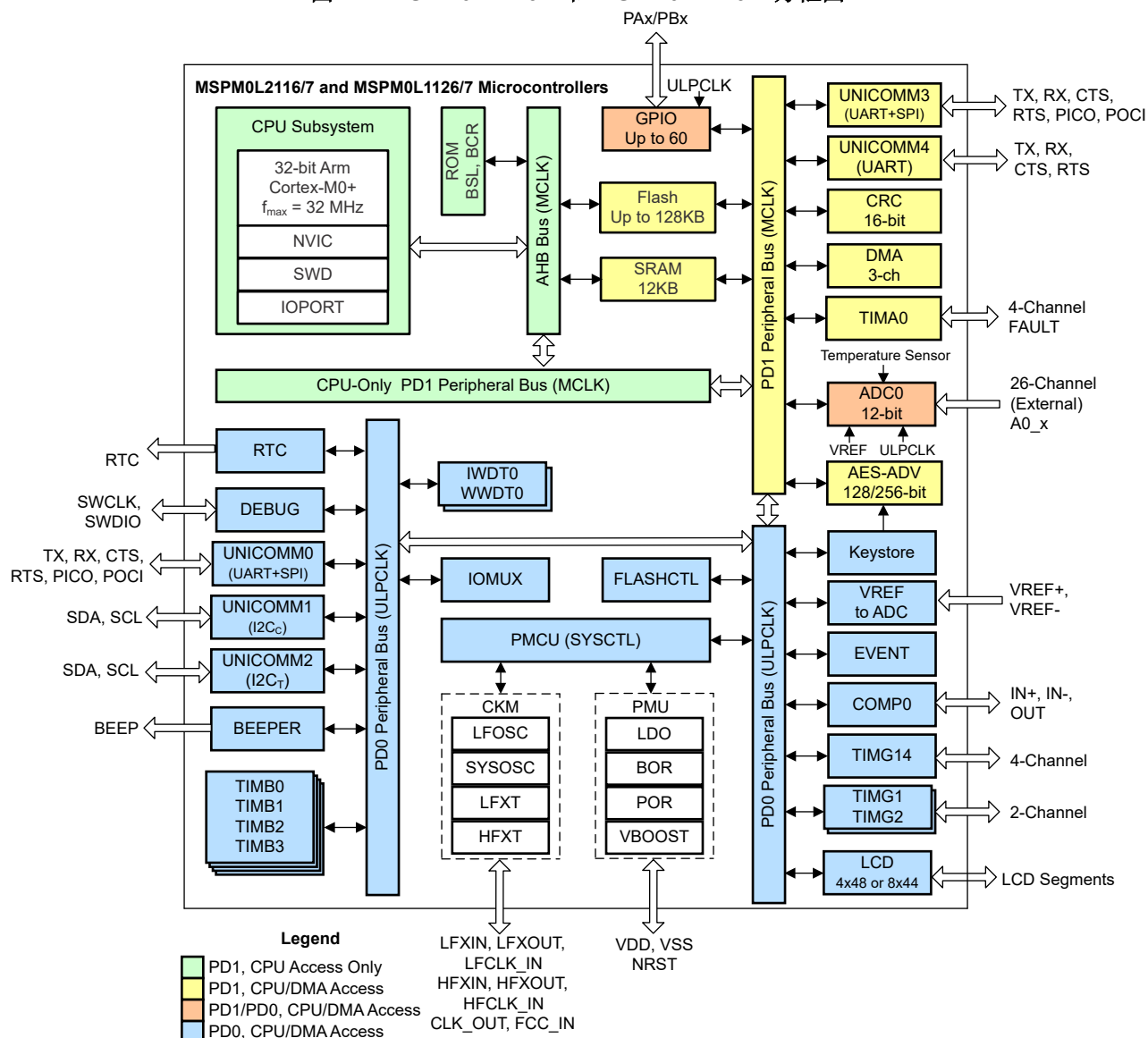
图 4-1. MSPM0L2116/7 和 MSPM0L1126/7 方框图
